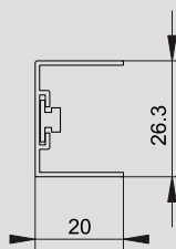
Endstab Anschlagsschiene mit Magnetleiste
